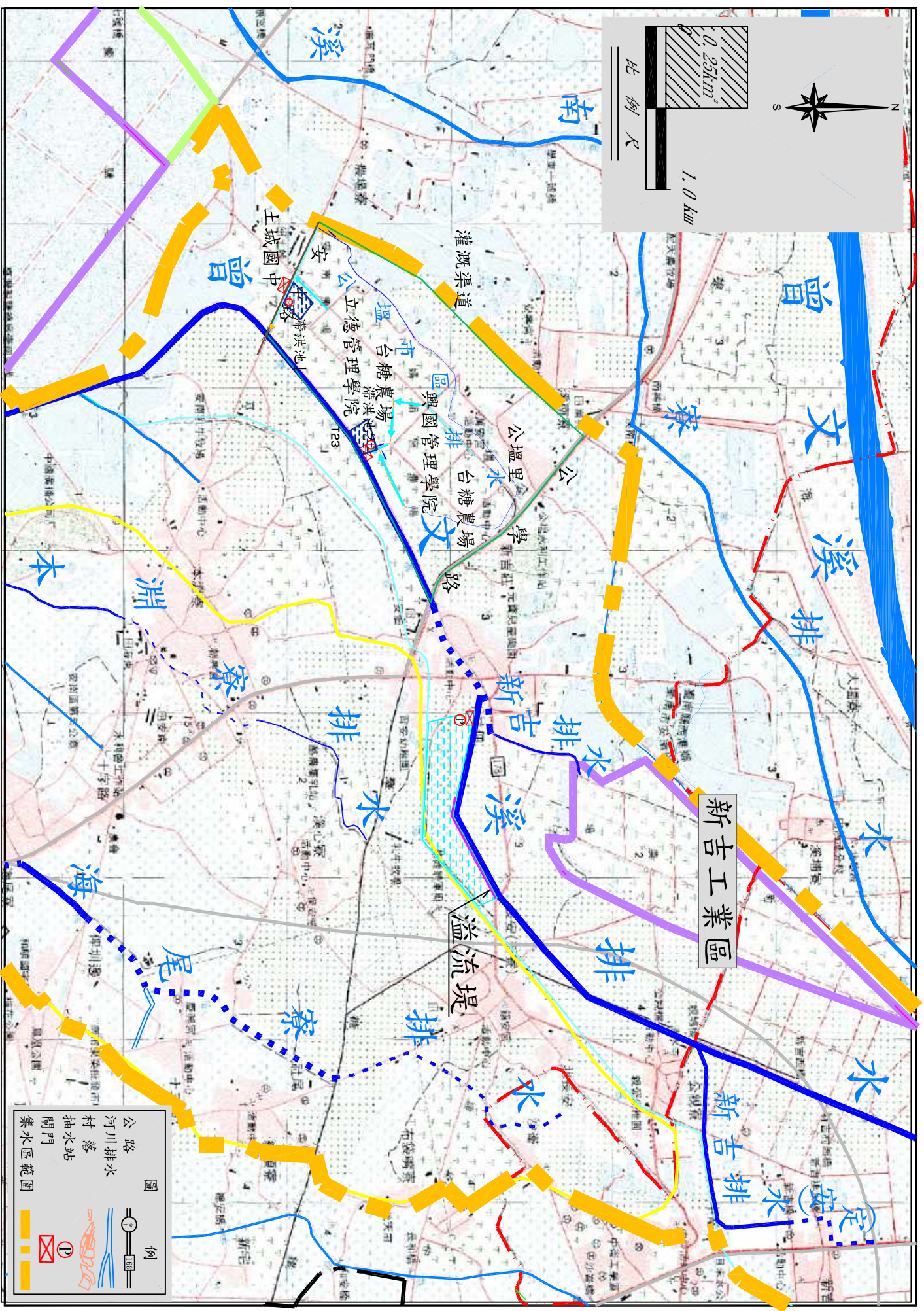
圖 7.1 台南地區曾文溪排水滯洪池案工程分佈圖
