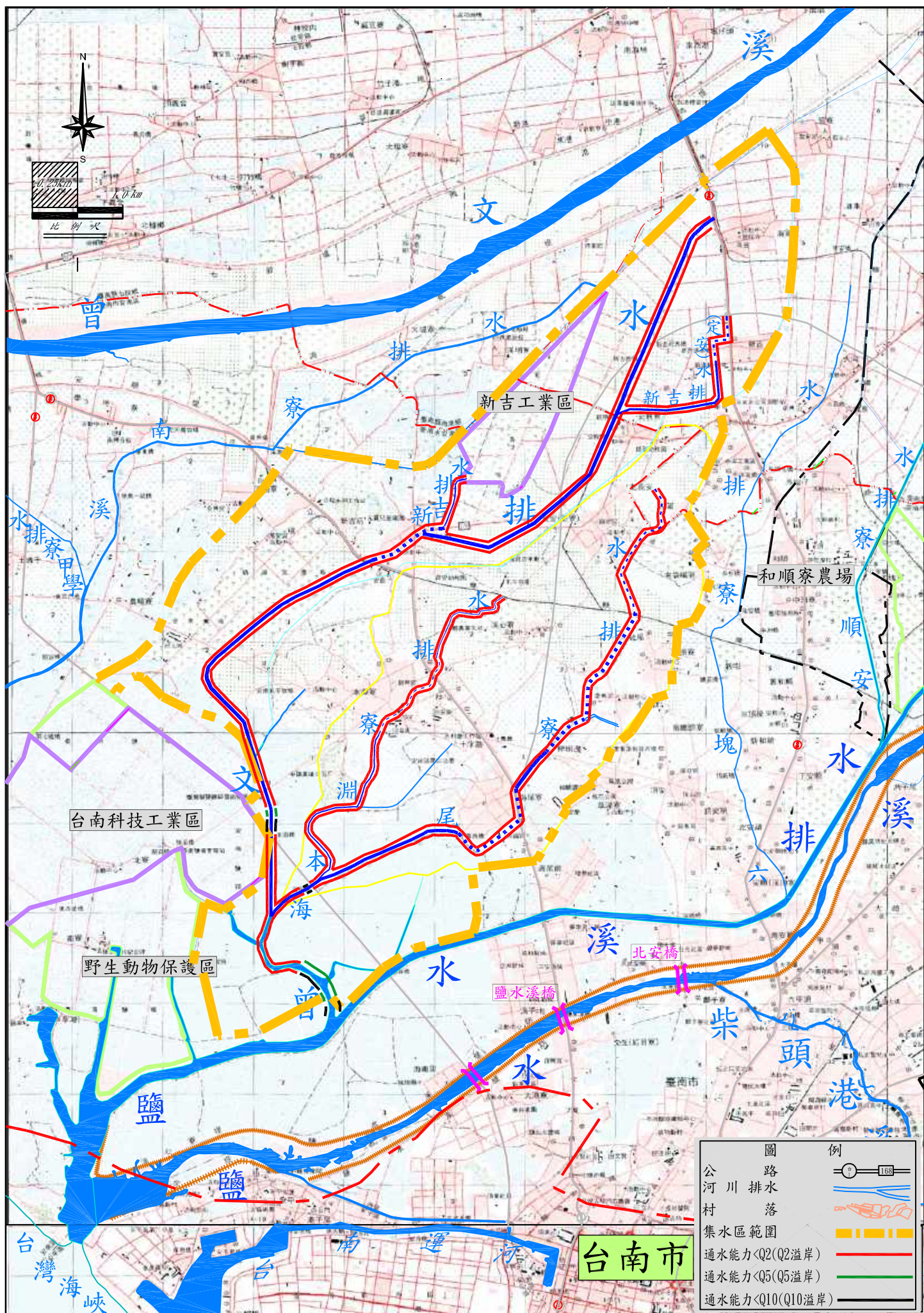
圖5.1 曾文溪排水現況通水能力示意圖
