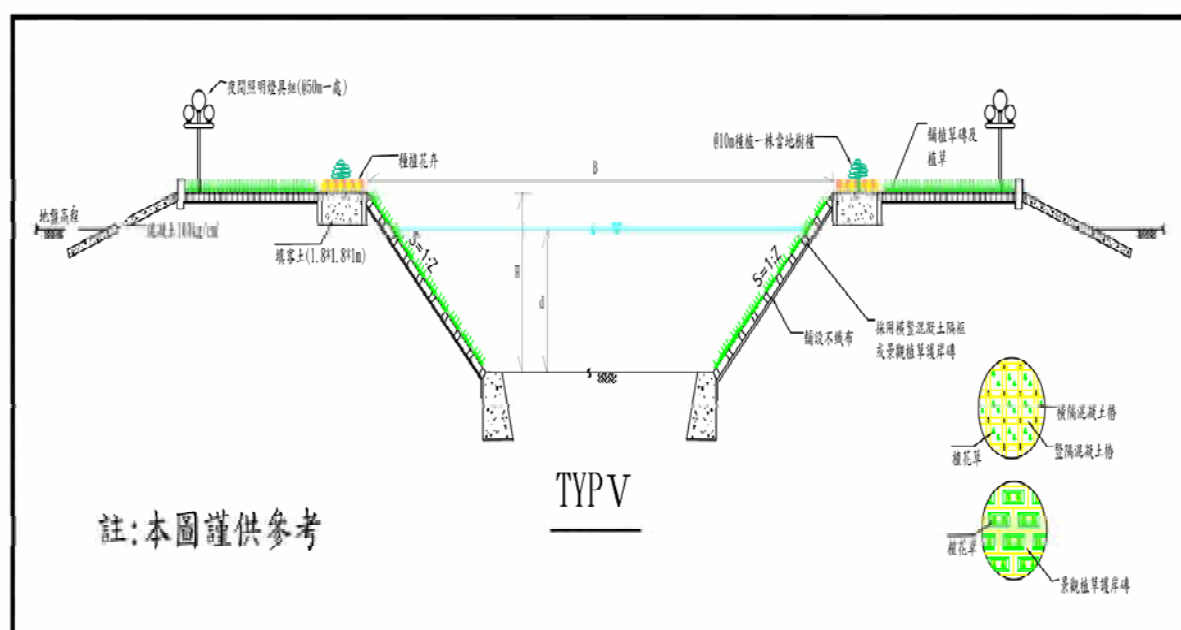
圖8.3 排水路規劃橫斷面示意圖
