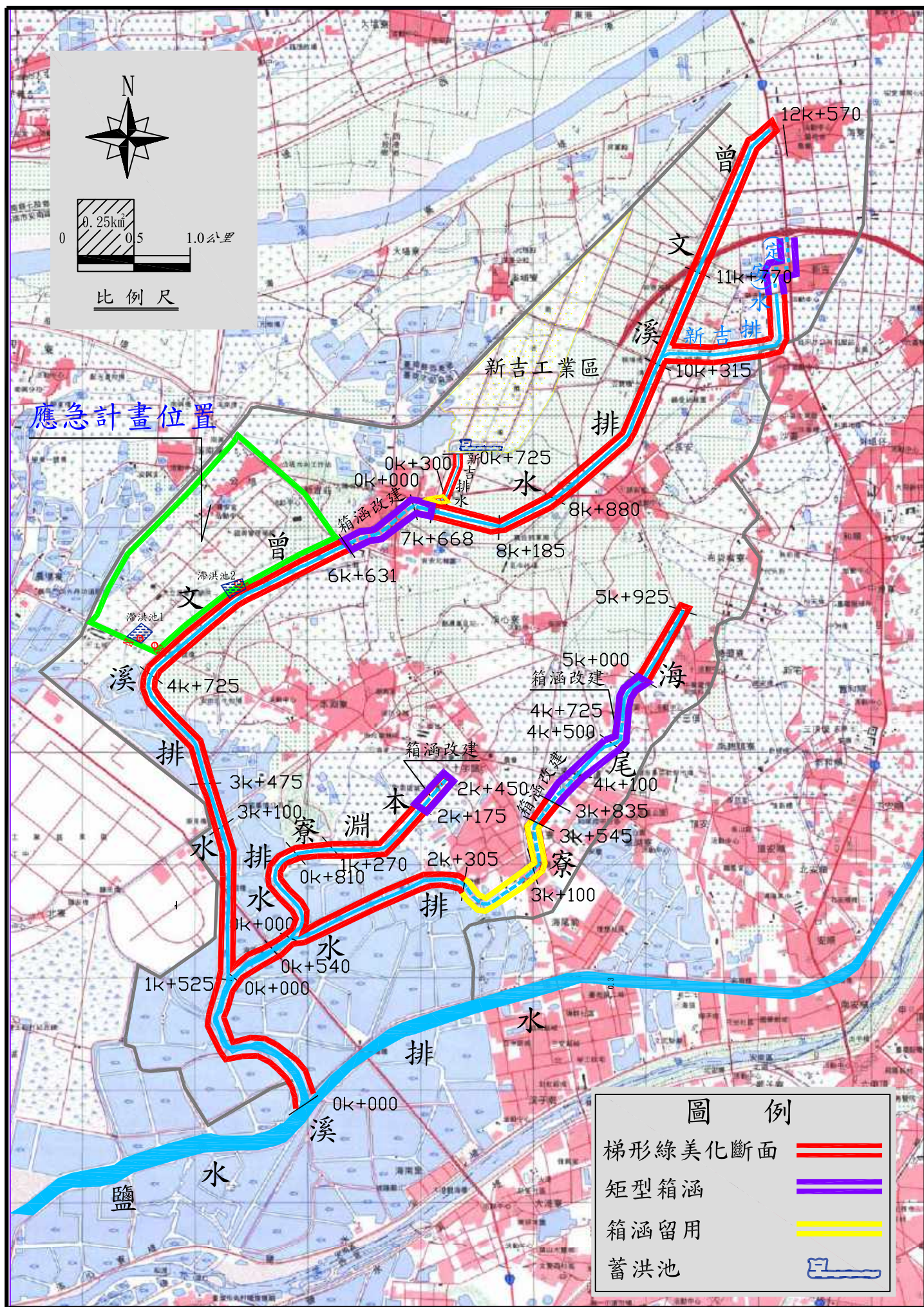
圖9.1 曾文溪改善工程平面位置圖
